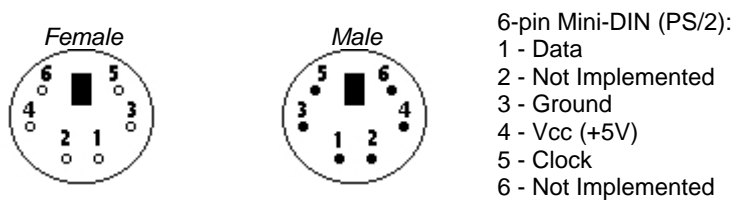
Gambar 2. Konektor PS/2 tipe 6 pin Mini-DIN
